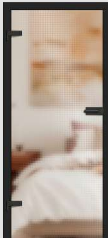
GRAF 69 POINT
